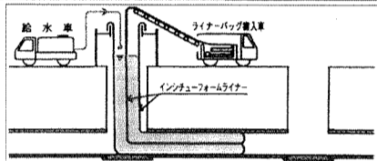
インシチューフォーム工法での管更新工事 場所/東部水路(美作市下香山地内) ・口径: 350mm ・長さ: 421m
